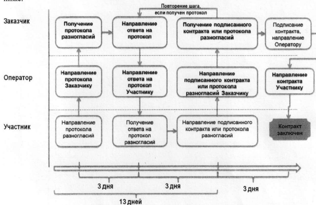
Рисунок 28. Алгоритм обмена протоколом разногласий при заключении контракта
